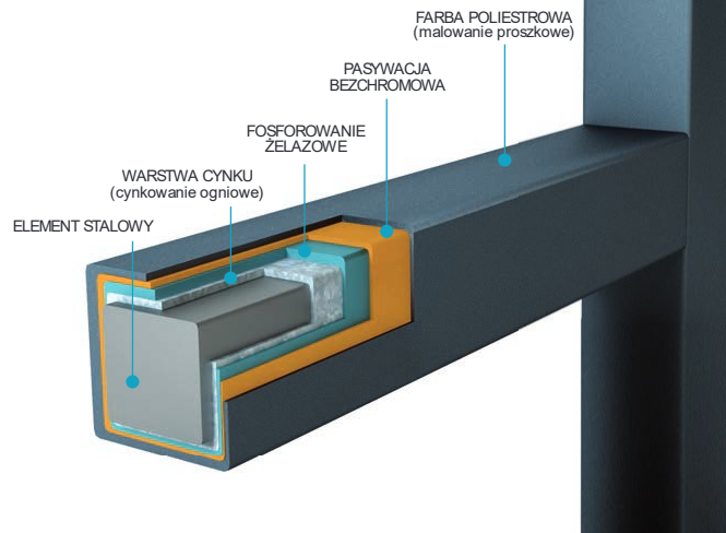
Przekrój przez element zabezpieczony w systemie DUPLEX
